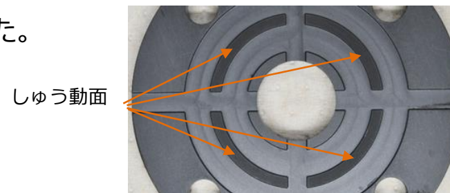
試験後の試験片しゅう動面と試験軸の外観
