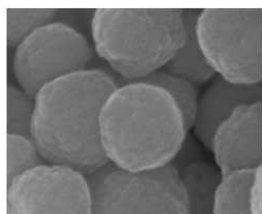
球状( \text{Fe}_3\text{O}_4 )
