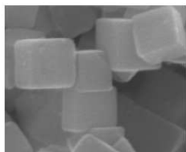
六面体( \text{Fe}_3\text{O}_4 )
