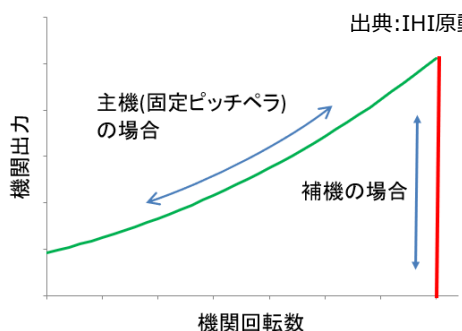
主機・補機における回転数・出力の関係(イメージ)
