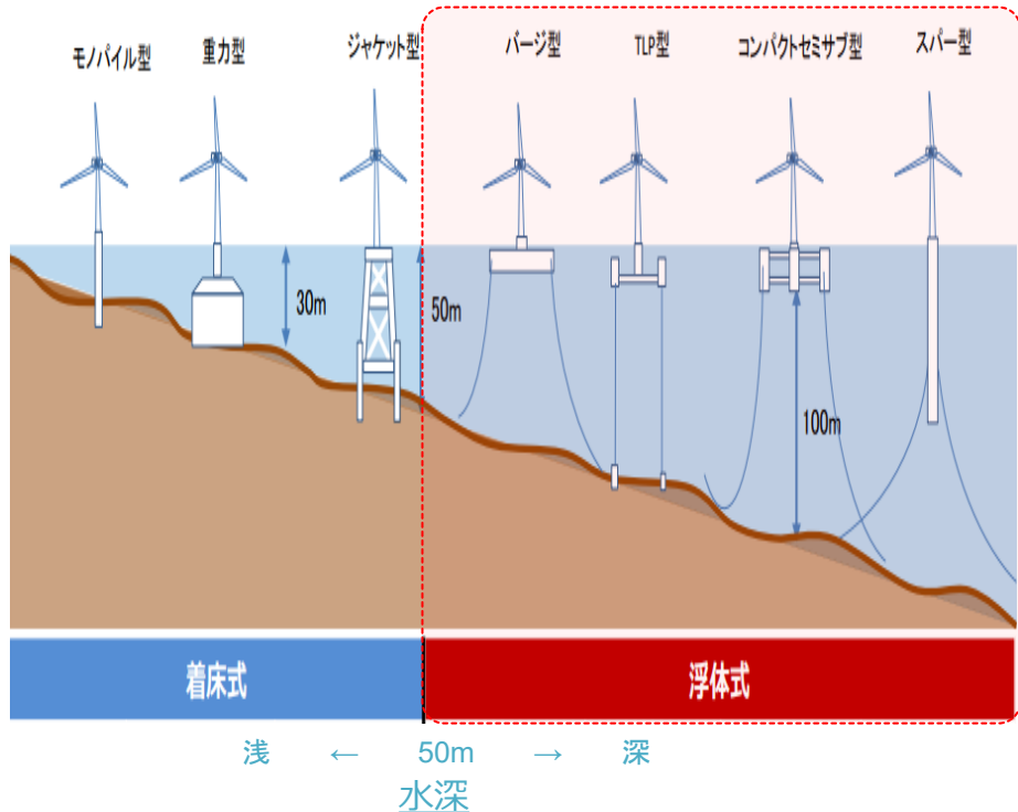
「洋上風力発電の低コスト化」プロジェクトの研究開発・社会実装計画(案)の概要 経済産業省 資源エネルギー庁より抜粋
